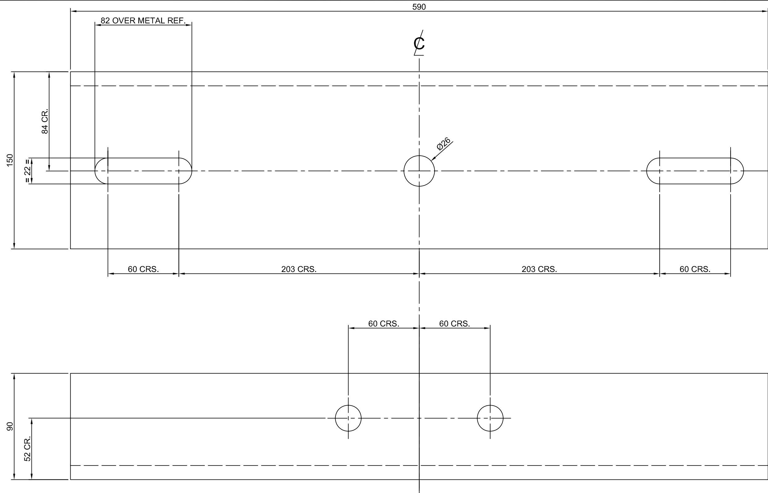
ITEM 7. 590 LONG x 150 x 90 x 12 THICK M.S. UNEQUAL ANGLE.
